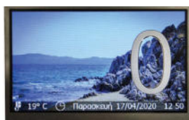
TFT 5 Farbbildschirm (Aufl.: B 480px, H 272px, Farbtiefe 24bits) Wi-fi Verbindung Stockwerk Nummer Uhrzeit - Datum Temperatur Richtungspfeile 2 Sprachen (Englisch - Griechisch)
