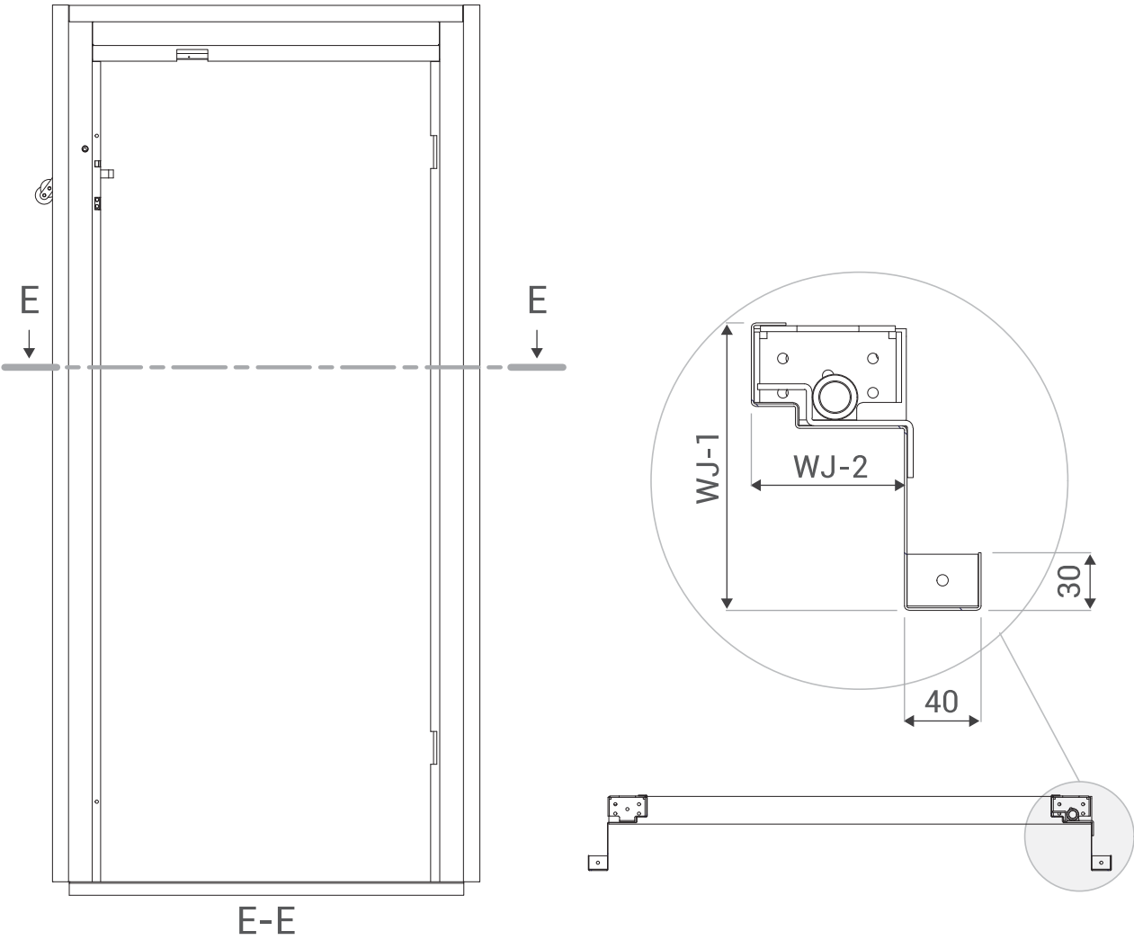
Frame with wall Jambs / Αγκαλιαστό Κάσωμα
